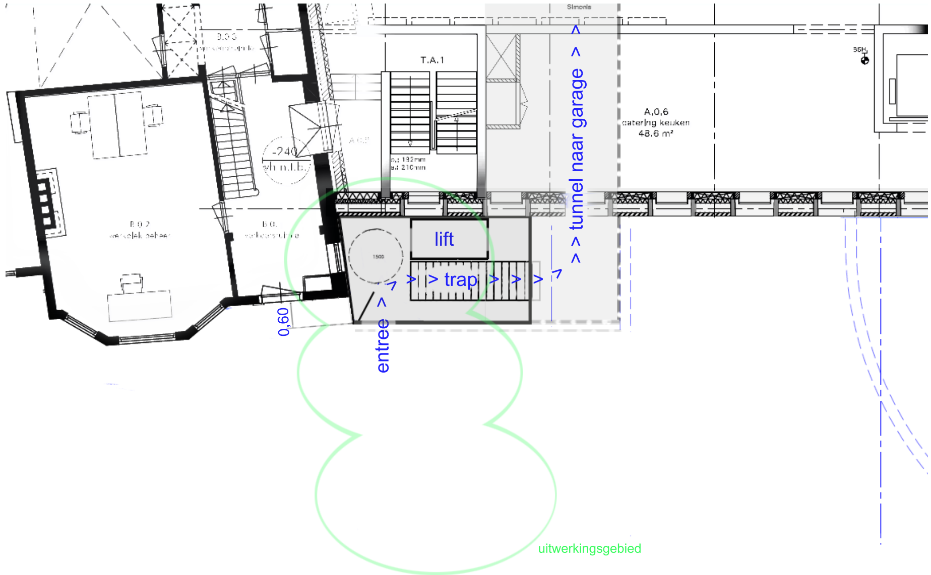
Variant 1. vrijstaand voor gebouw A
